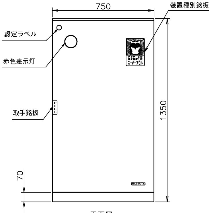
正面図
